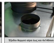
Έξοδοι θερμού αέρα έως και 4x140mm
